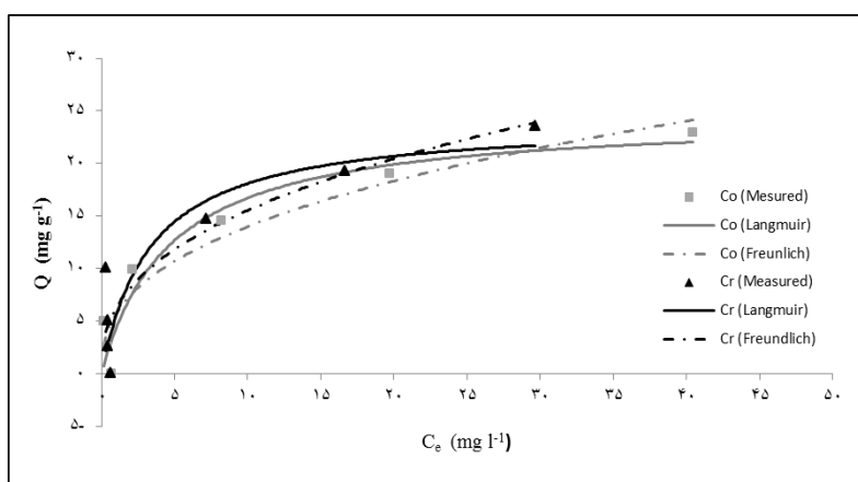
نمودار ۶- ایزوترم‌های جذب سطحی کروم و کبالت توسط نانو رس بنتونیت
