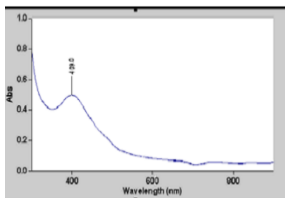
شکل ۲- طیف سنجی قابل مشاهده-فرابنفش نانوذرات نقره تشکیل شده از عصاره گل اکالیپتوس کامالدولنسیس تایید سنتز نانوذرات با روش طیف سنجی مادون قرمز
